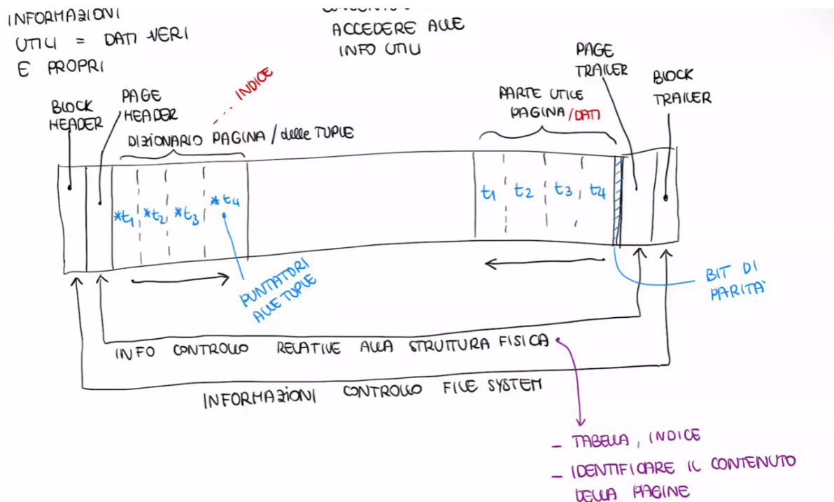
Figura 105: Struttura pagina
