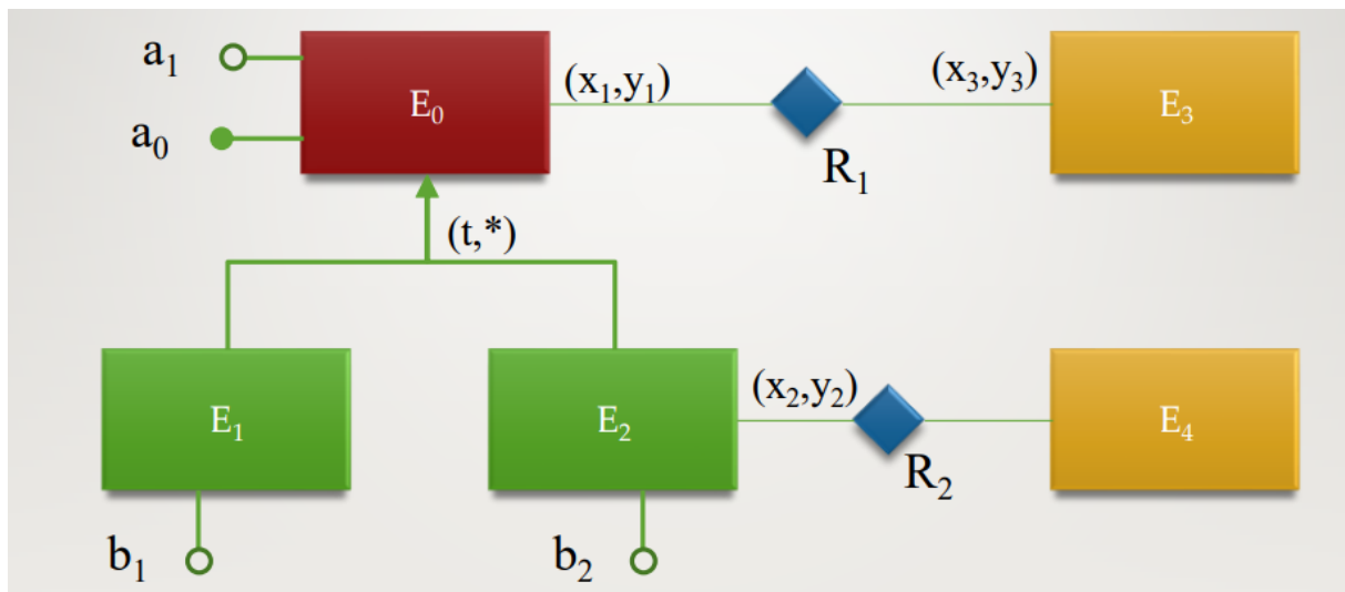
Figura 28: Schema iniziale
