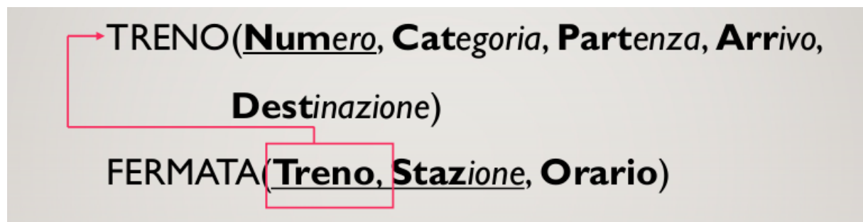
Figura 71: Progettazione Logica
